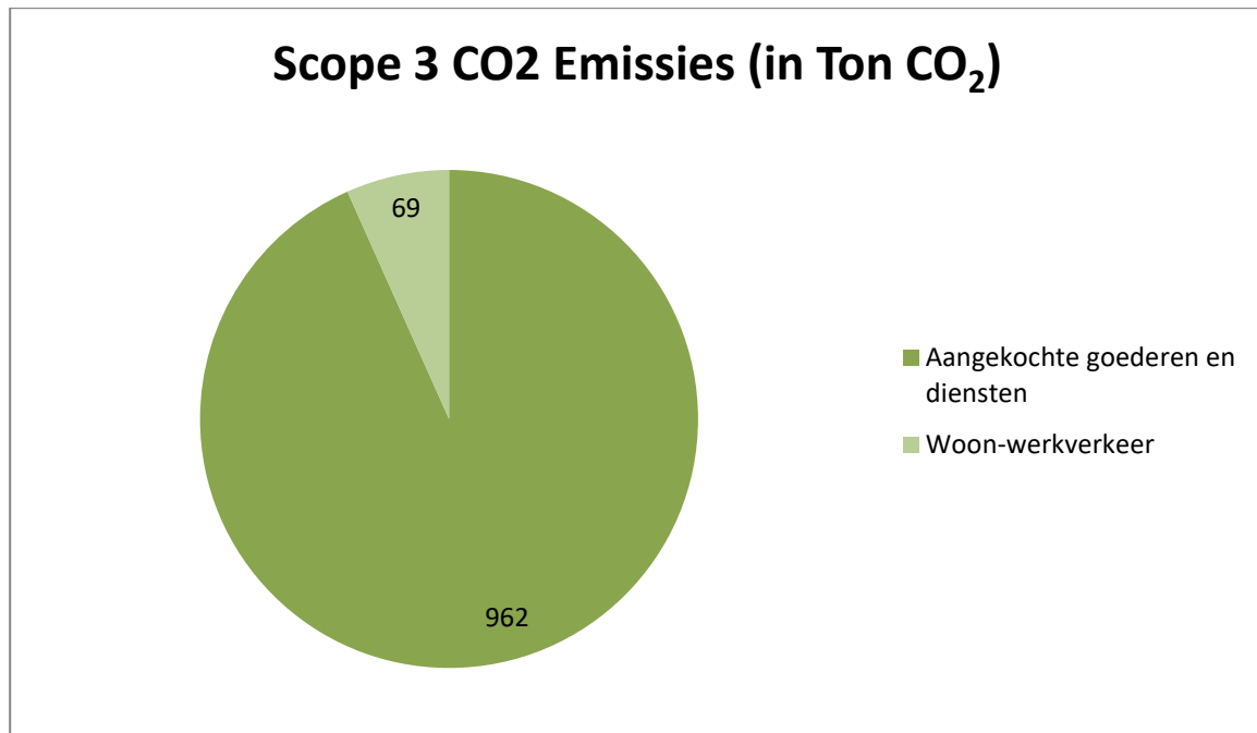
Grafiek 1: Scope 3 CO 2 Emissies jan-jun 2017 (in Ton)
